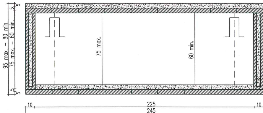
SEZIONE LONGITUDINALE
