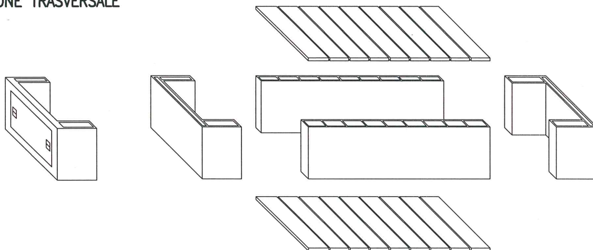
ESPLOSO ASSONOMETRICO
