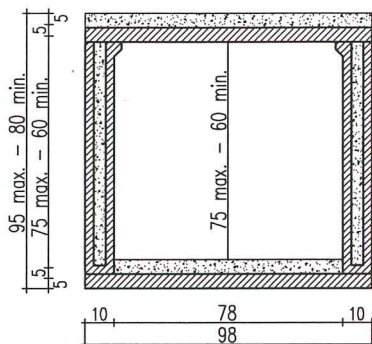
SEZIONE TRASVERSALE
